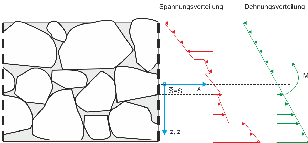
Abbildung 35: Spannungs- und Dehnungsverteilung am Längsschnitt eines mörtelvergossenen Schuttsteindeckwerks.
