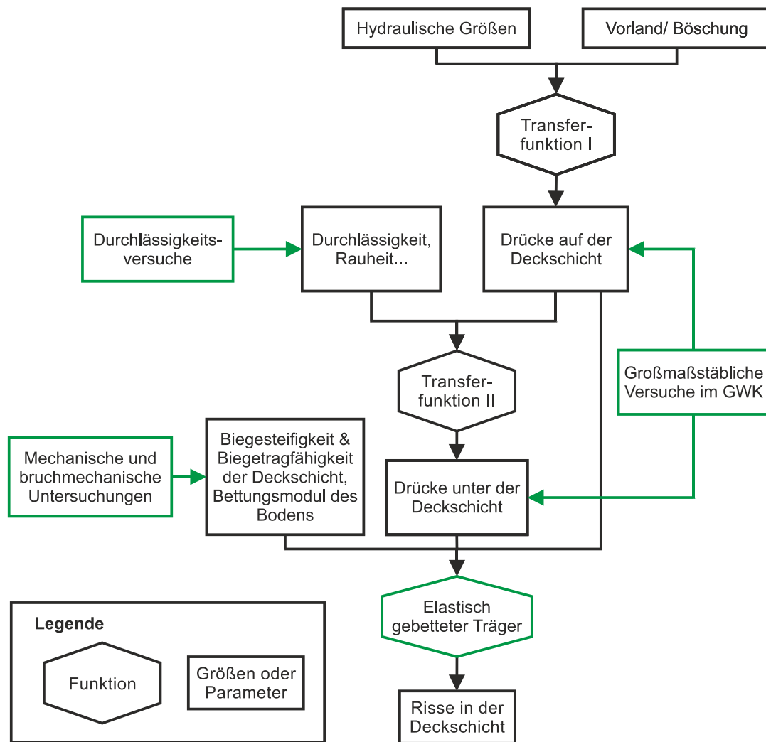
Abbildung 31: Verwendete Modelle, Größen und Parameter zur Beschreibung der Rissbildung in der Deckschicht (Prozesskette verändert nach Groot et al. 1988) und eigene Untersuchungen im HYGED-Projekt (grün umrandet).
