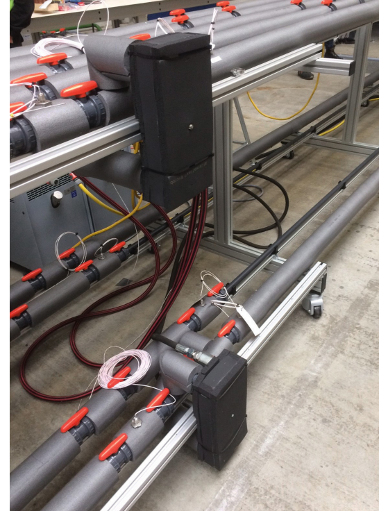
Opstelling van het drinkwaterdistributienetje in het laboratorium.
