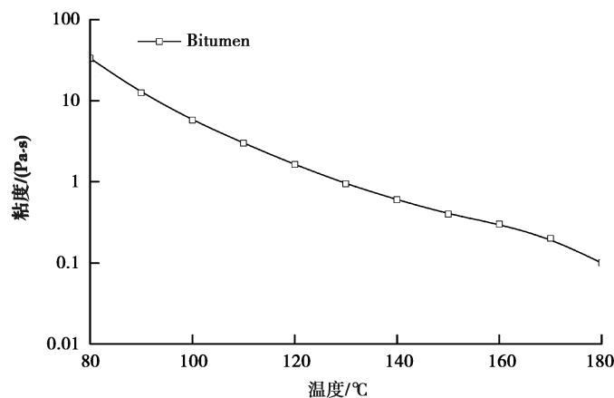
图2 基质沥青粘度随温度的变化曲线
