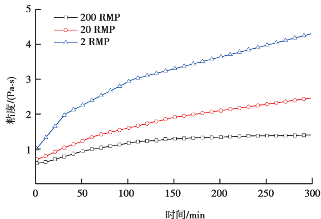
图 4 稀释环氧沥青 EB25 在不同剪切速率的粘度变化曲线
