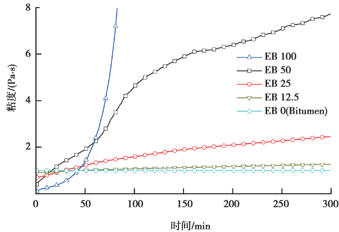
图 3 不同稀释比的环氧沥青的粘度变化曲线
