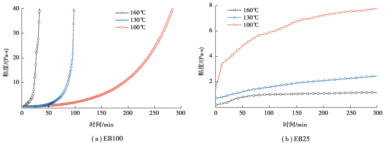
图1 环氧沥青在不同固化温度下的粘度变化曲线
