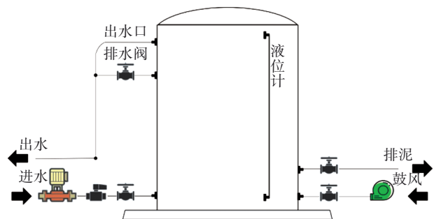
图1 中试反应器示意
