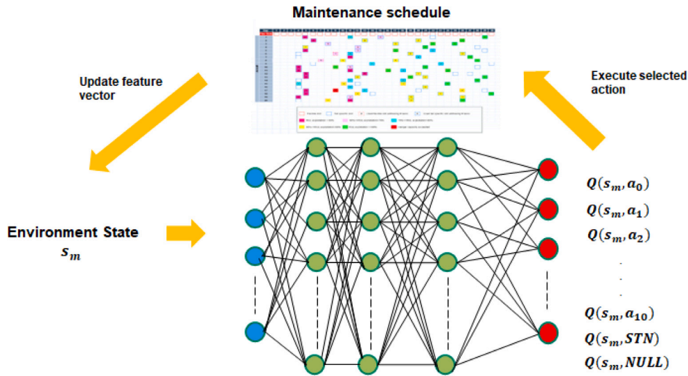
Fig. 5. DQN structure.
