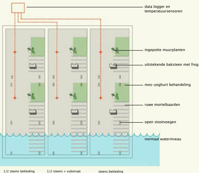
Basisopbouw panelen proefopstelling. Bron: TUD.
