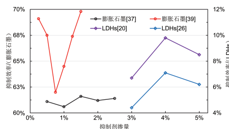
图 8 层状材料对 VOCs 的减排效果对比 [20,26,37,39] (电子版为彩图)
