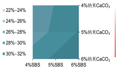
图 15 不同百分比的纳米 CaCO 3 /SBS 复合抑制剂的减排效果 [25]
