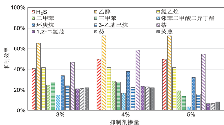
图9 LDHs 对各 VOCs 分子的选择性抑制 [41]
