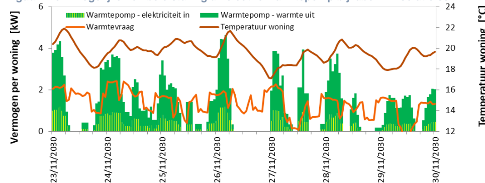
Figuur 12c Mogelijke flexibele sturing all-electric warmtepomp bij label A+ isolatie schil
