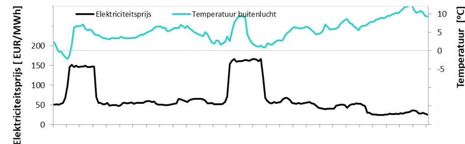
Figuur s3a: Elektriciteitsprijs en buitentemperatuur tijdens winterweek 2030 (weerjaar 2015)
