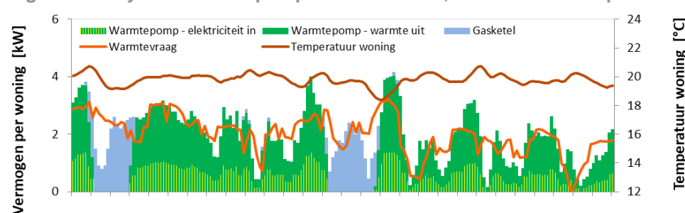
Figuur B9 : Hybride warmtepomp label B isolatie, 4kW netwerkcapaciteit
